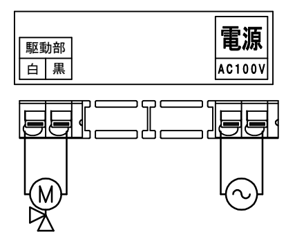
端子結線図
