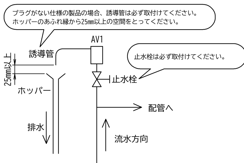
図2 配管例
