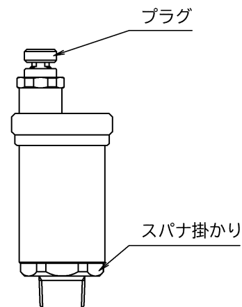
図1 製品外観
