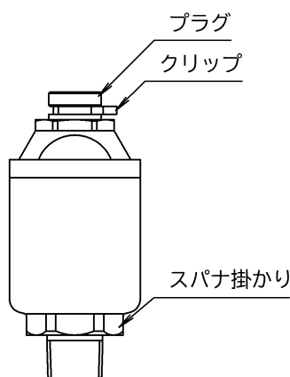
図1 製品外観
