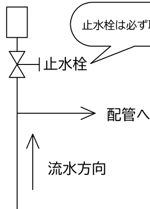
図2 配管例
