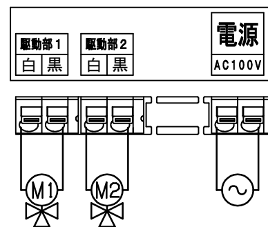
端子結線図
