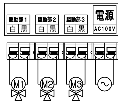
端子結線図
