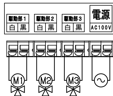
端子結線図
