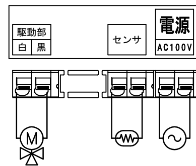
端子結線図
