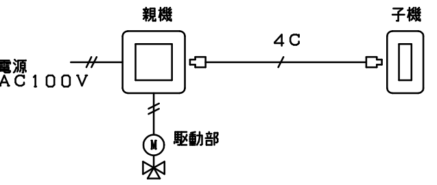
配線図
