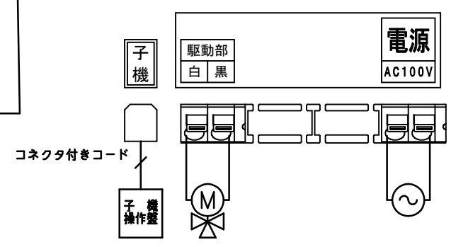
端子結線図
