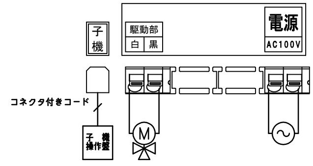
端子結線図
