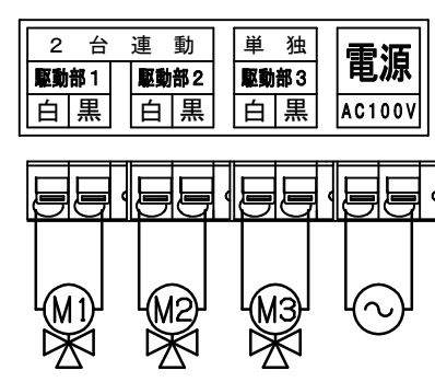
端子結線図
