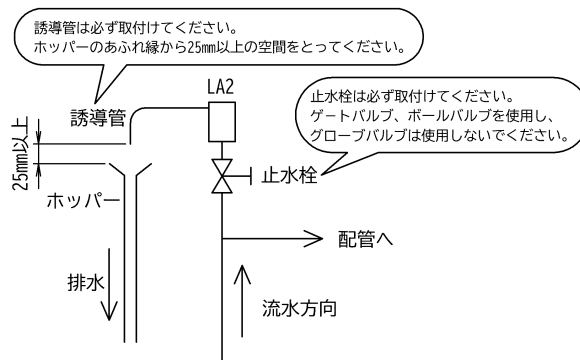
配管例
