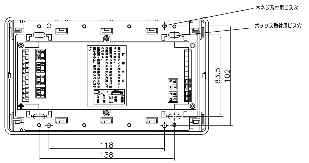
外形寸法図
