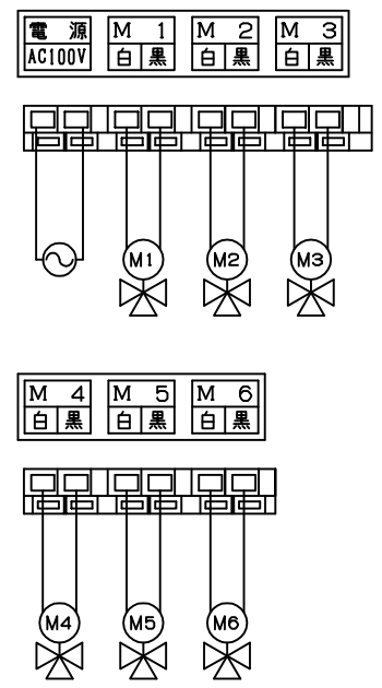
端子結線図
