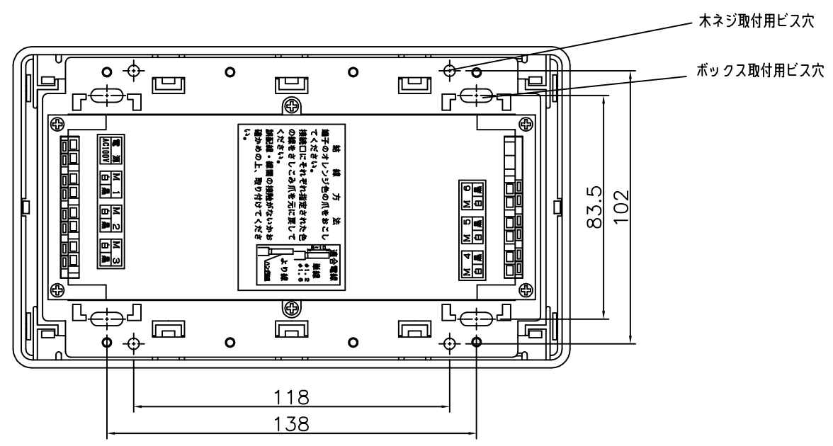
外形寸法図
