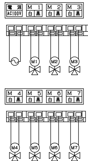
端子結線図
