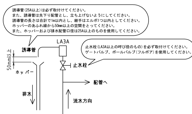
図3 配管例2
