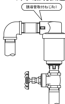
図2 配管例1
