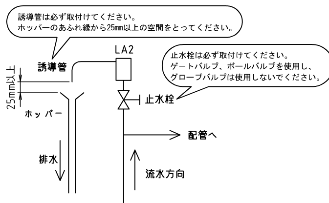
配管例
