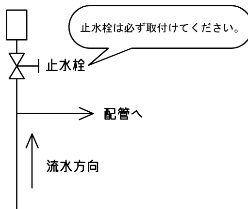
配管例
