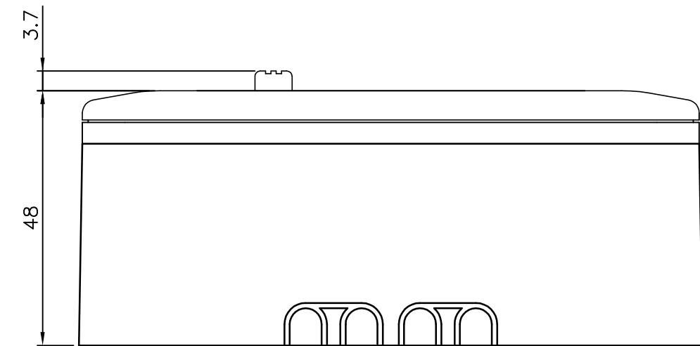
外形寸法図
