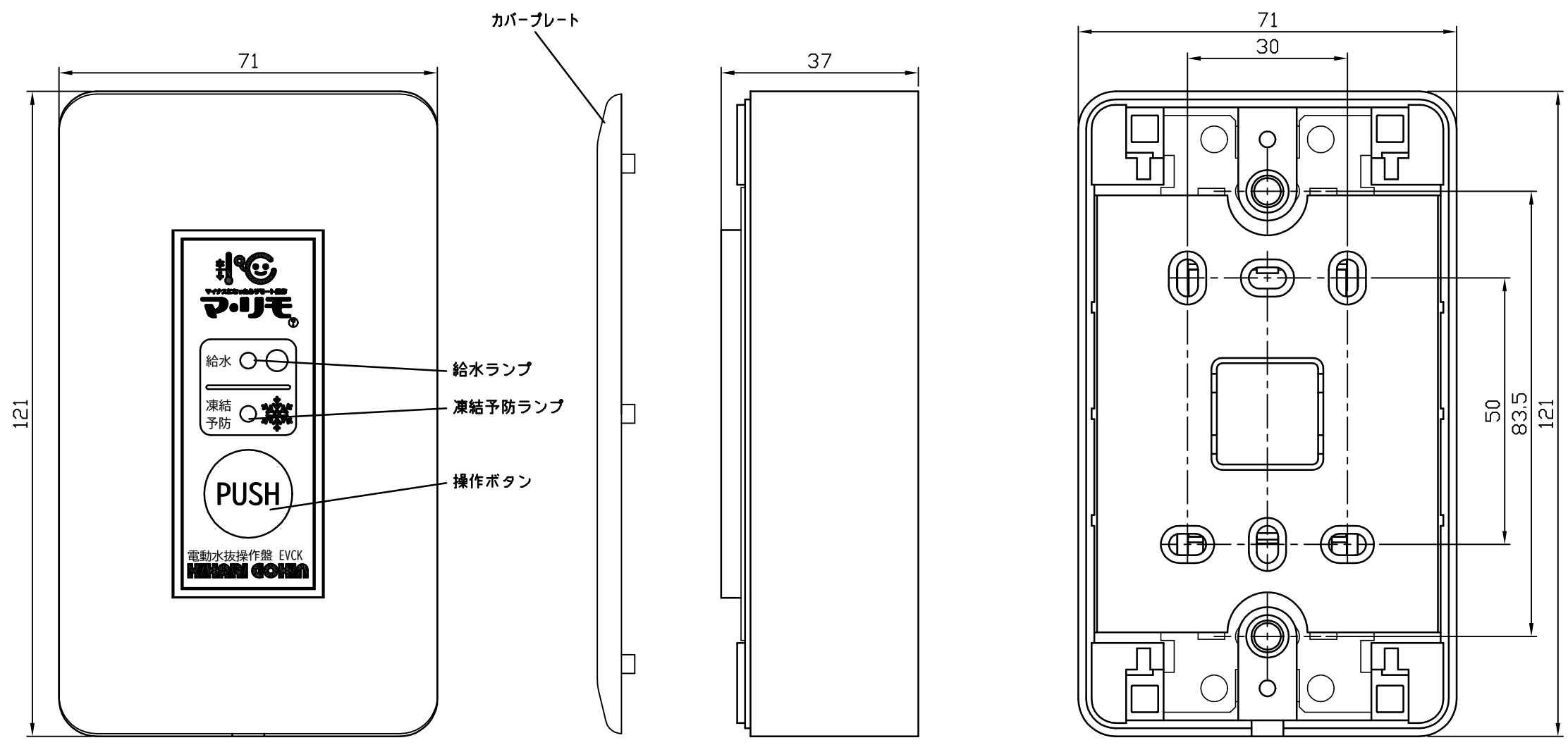
子機外形図
