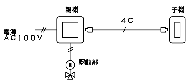
配線図
