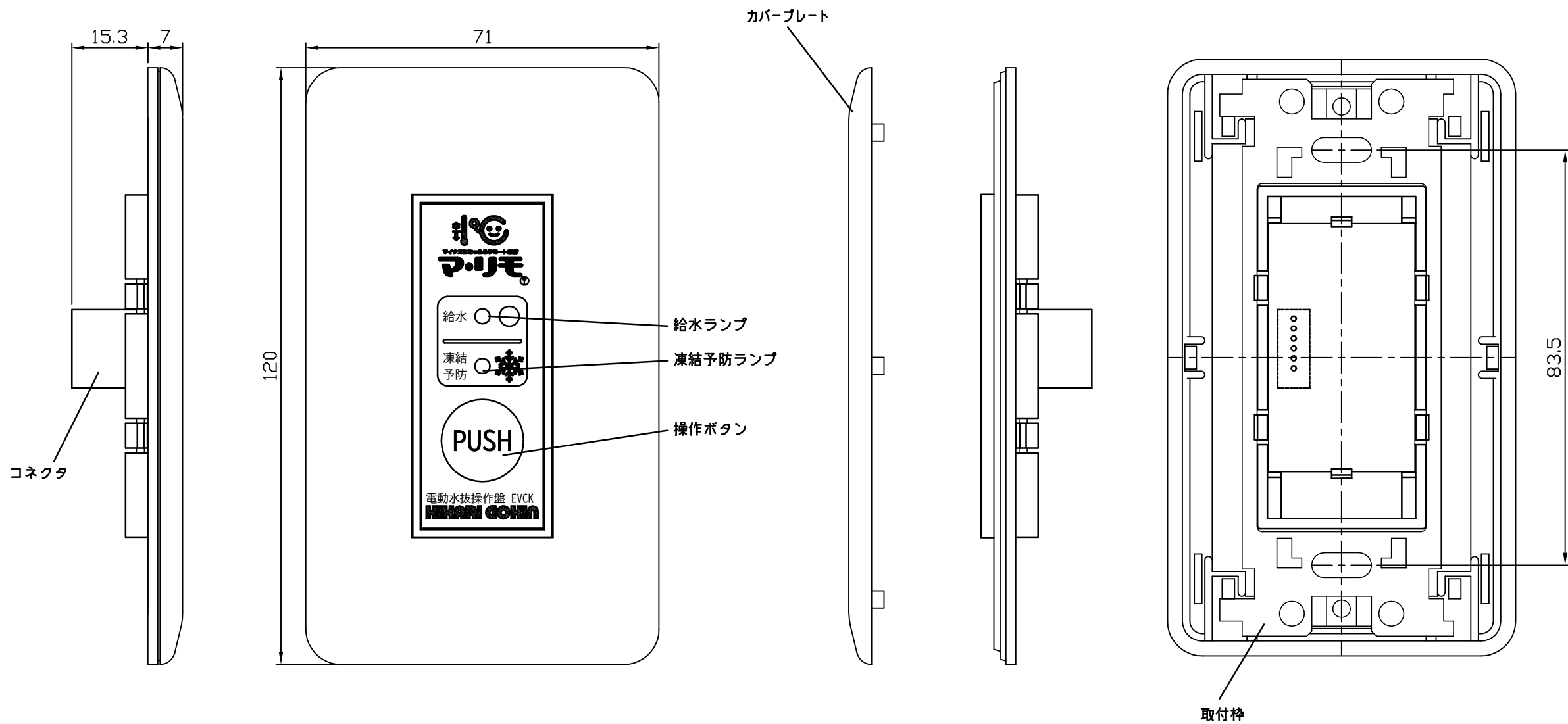
子機外形図
