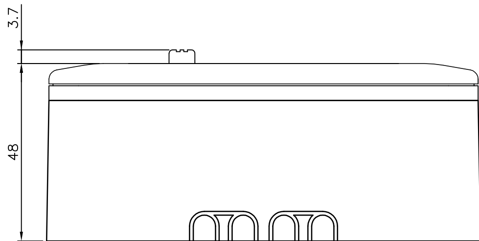
外形寸法図
