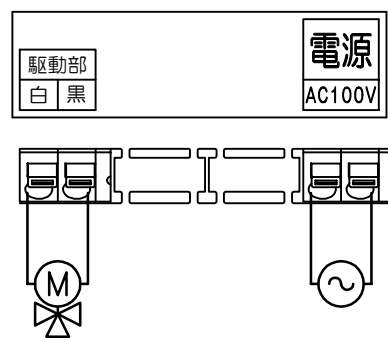
端子結線図
