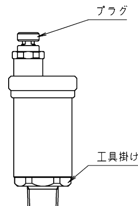
図1 製品外観
