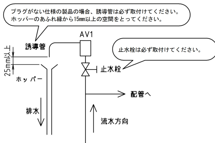
図2 施工例
